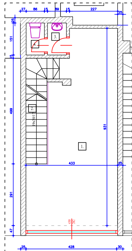
OSNOVA PRIZEMLJA LOKALA 4
