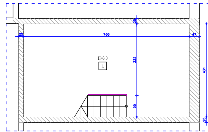
OSNOVA PODRUMA LOKALA 4
