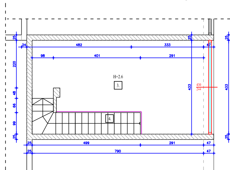
OSNOVA I SPRATA LOKALA 4
